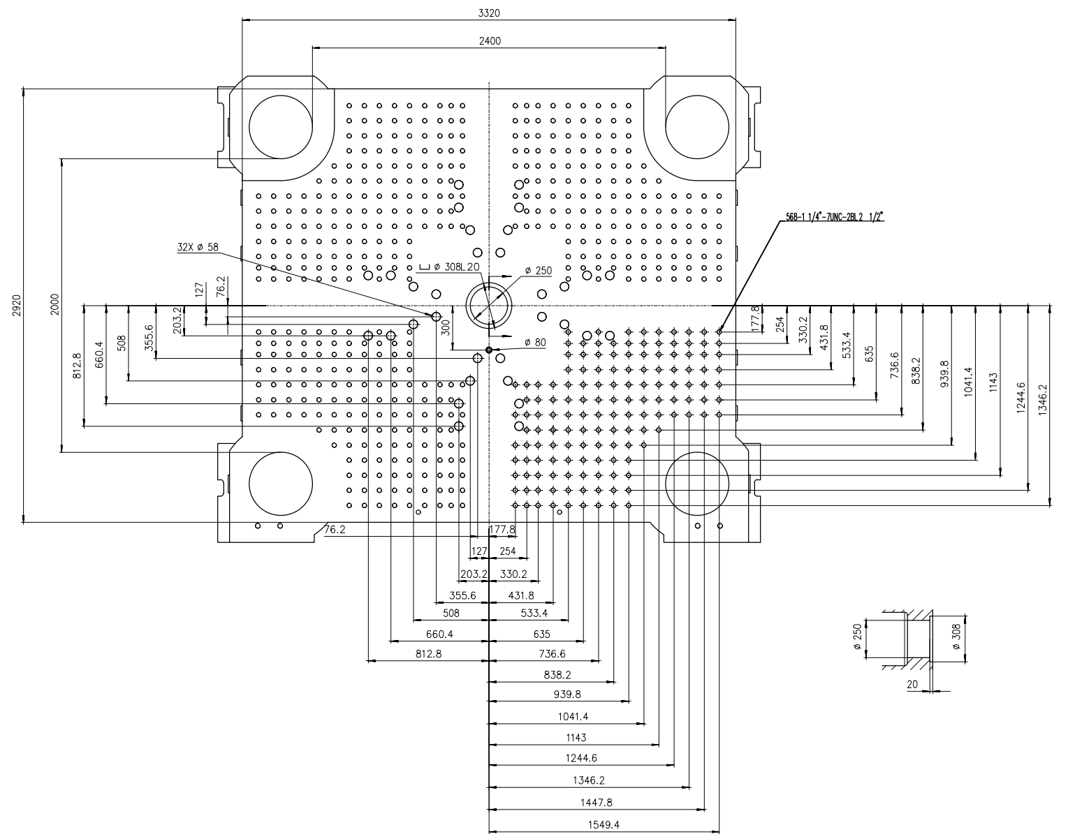
Moving Platen
