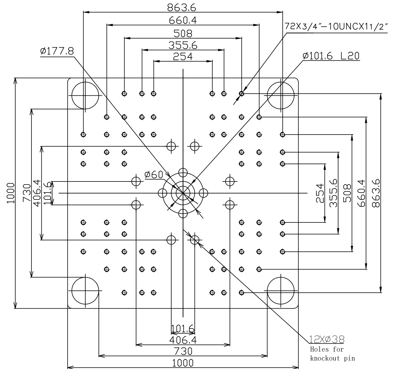
Moving Platen
