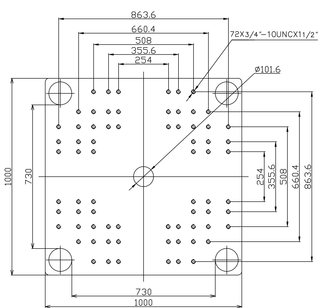
Fixed Platen
